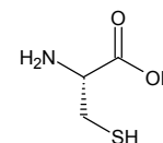
L-Cysteine
