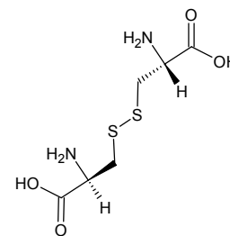
L-Cystine
