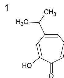
Hinokitiol
