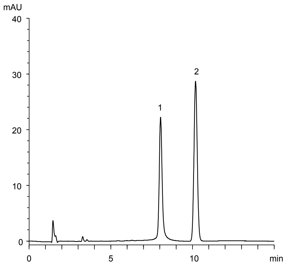
Hinokitiol
